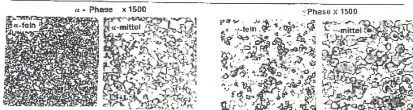
Hartmetall — Metallographische Bestimmung des Mikrogefüges
